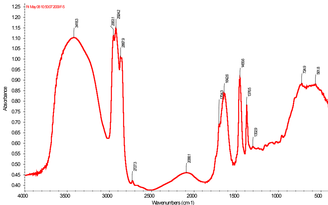
Сурет 5 — F5 үлгісінің ИҚ-спектрлері (шыңмен).
