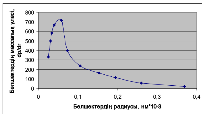
Сурет 2 — Бөлшектердің мөлшеріне байланысты таралуы
