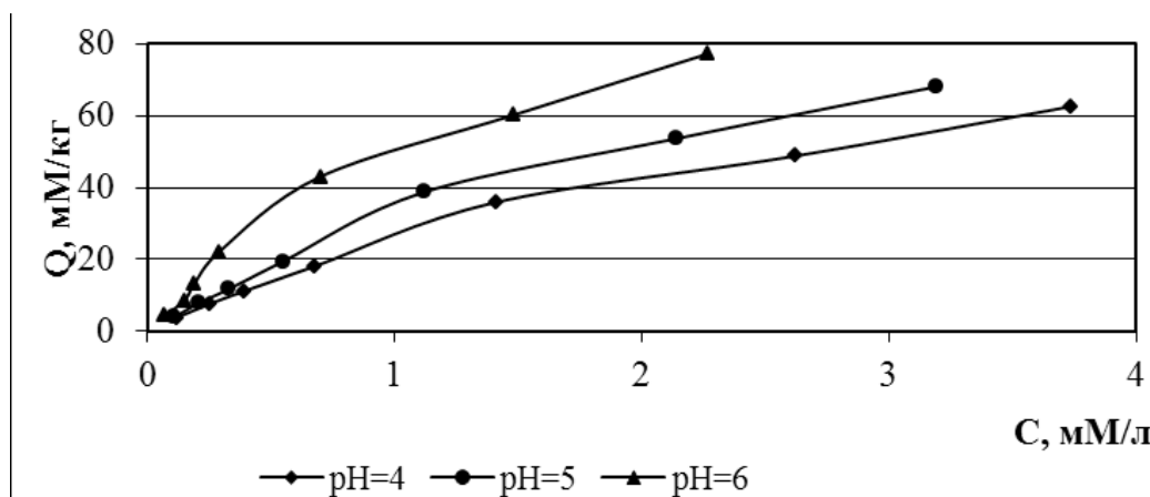
Рис. 3. Изотермы поглощения свинца почвой
