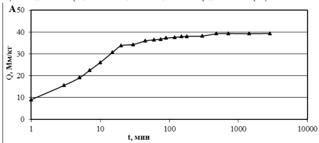
Рис. 1. Динамика поглощения свинца почвами
