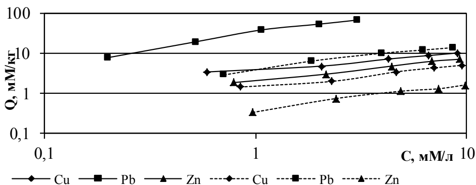
Рис. 4. Изотермы поглощения ТМ почвой при моно- и полиэлементном загрязнении ( — — моноэлементное загрязнение; - - - - - полиэлементное загрязнение)
