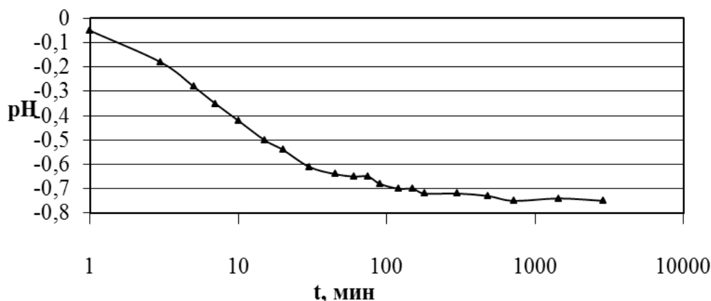
Рис. 2. Динамика изменения pH в процессе поглощения свинца почвой
